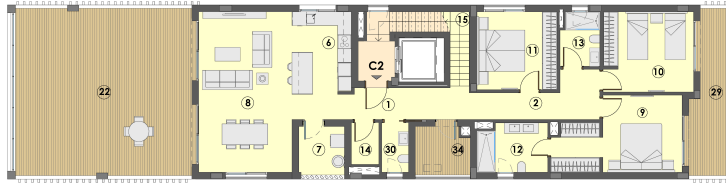
PLANTA SEGUNDA
