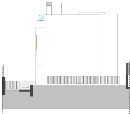
Alzado Norte
