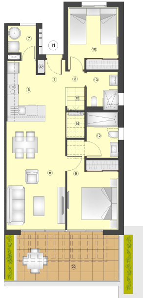
PLANTA PRIMERA
