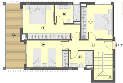
PLANTA PRIMERA
