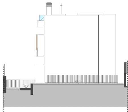
Alzado Norte
