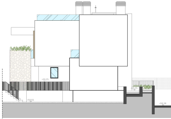
Alzado Este
