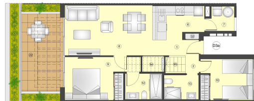
PLANTA TERCERA
