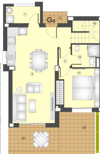
PLANTA BAJA
