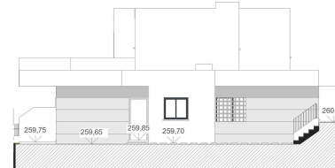
ALZADO SUR
