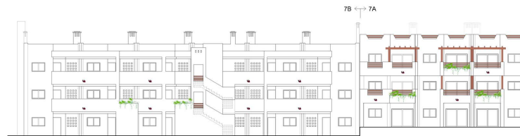
ALZADO POSTERIOR NORESTE
